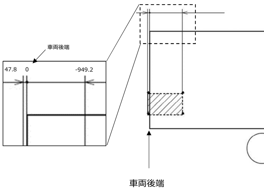
図5（側面視）
