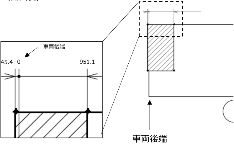
図3（側面視）
