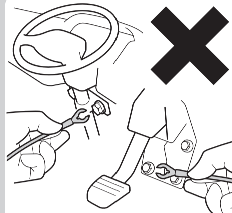
車体からアースを取得する場合はステアリングやブレーキ系統のボルトを使用しないこと
