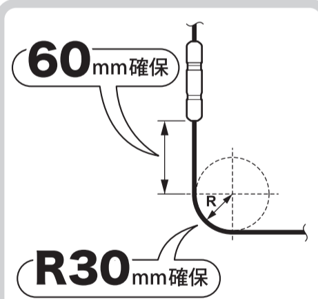
コネクター付近でケーブルを屈曲させないようにすること(コネクター端末から60mm程度の直線部分を確保)ケーブルに曲げを伴う場合は、最低30mm程度の曲げRを確保すること(無理な屈曲は避けること)
