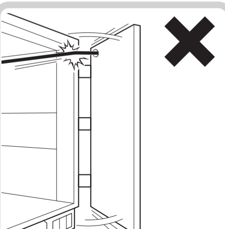
配線経路上の摺動部には余長を確保し、ケーブルの引っ張りや圧縮を避けること
