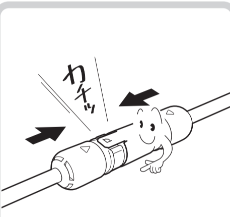
コネクター接続時は嵌合音やクリック感を確認して、確実に接続すること
