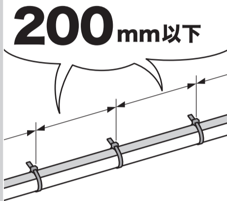
ケーブルの固定は200mm以下の間隔を目安に固定すること
