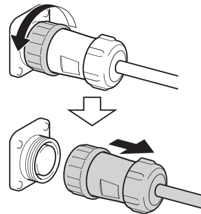
ダイヤル付きコネクターの脱着は、ダイヤル部分を回転させてからまっすぐ引き抜くこと
