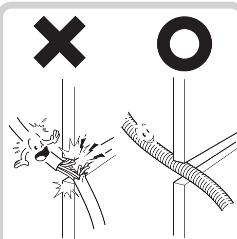
車両部品への噛みこみや強接触、干渉は避けること(やむを得ない場合はコルゲートチューブ等を使用してケーブルを保護すること)
