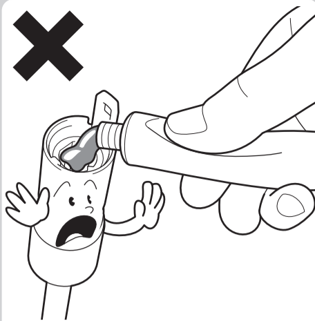
コネクター接続部にグリス等の異物を入れないこと
